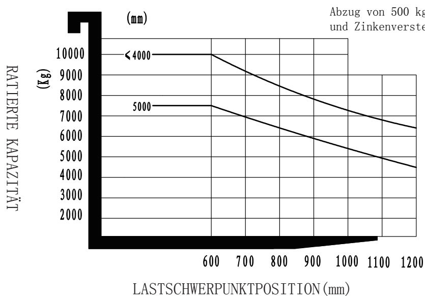
DIAGRAMM DER NENNKAPAZITÄTEN UND LASTSCHWERPUNKTE
